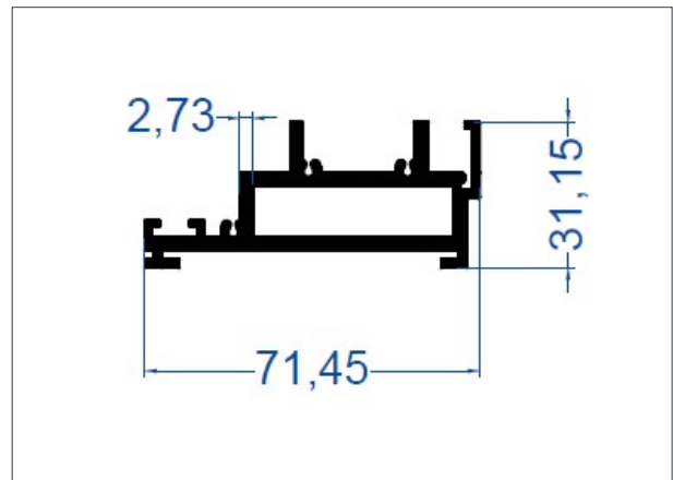
KASA PROFİLİ
