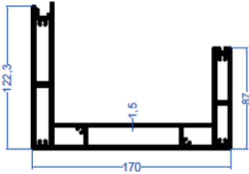
DERE PROFİLİ
