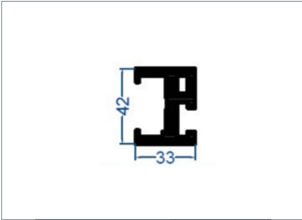
ÜST RAY
