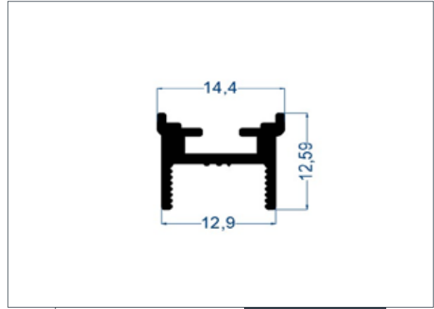
8 mm KANAT PROFİLİ
