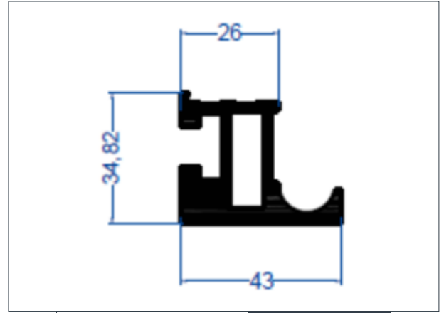
ÜST RAY
